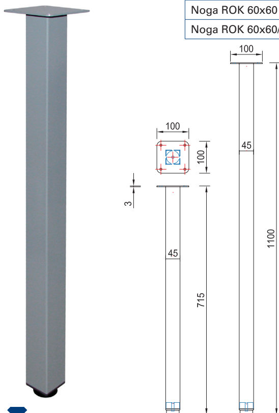
Noga ROK 45x45
