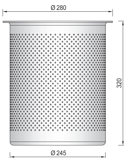
Koš za papir Ø245 mm, perforacija Ø3 mm
