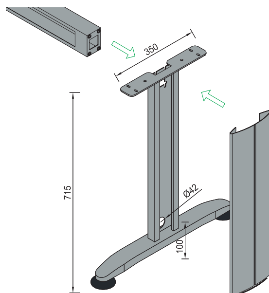
Sestav noge TAYA
