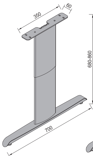
IRENA PLUS 700 konf.
