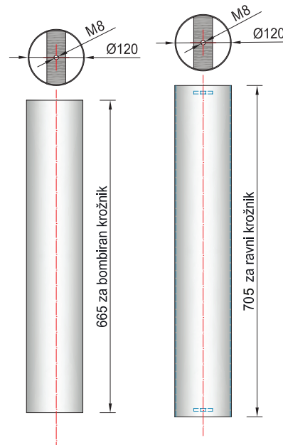
Steber noge MAX Ø120
