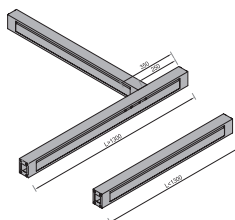
Vezniki pohištenih nog 19
