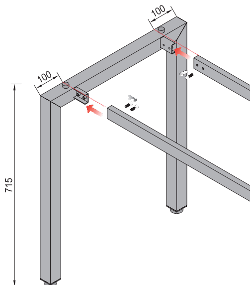
Sestav noge MIHA PLUS
