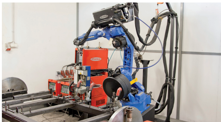
Ročno in robotsko varjenje MIG-MAG + TIG postopek
