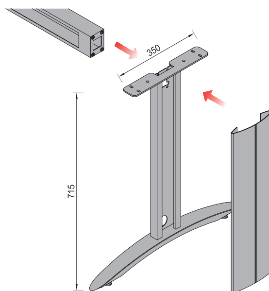
Sestav noge KIM
