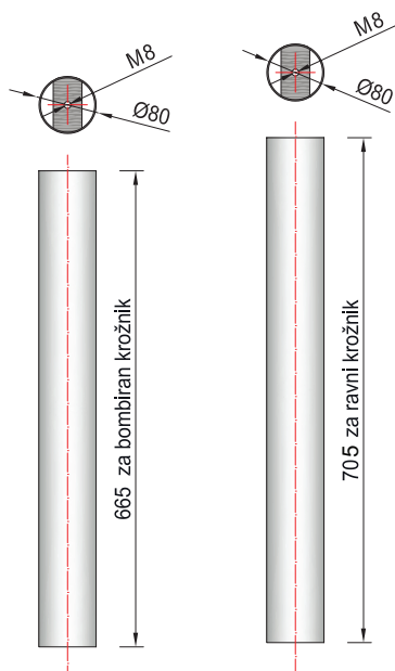
Steber noge MAX Ø80
