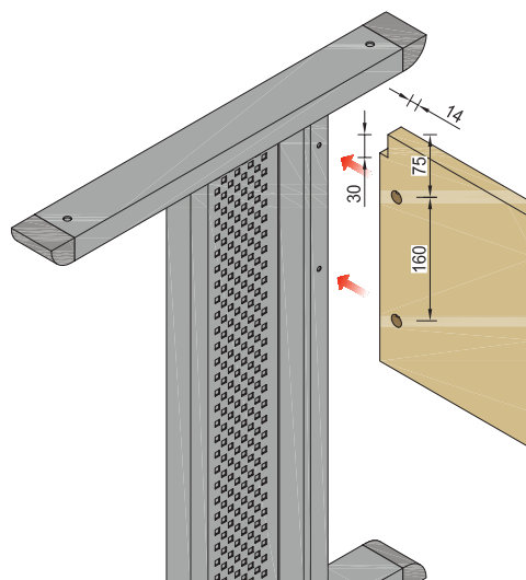
Sestav noge DONA PLUS
