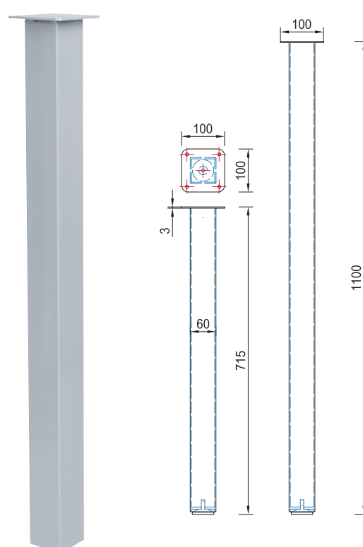
Noga ROK 60x60
