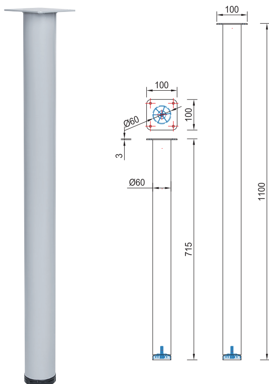
Noga ROK Ø60
