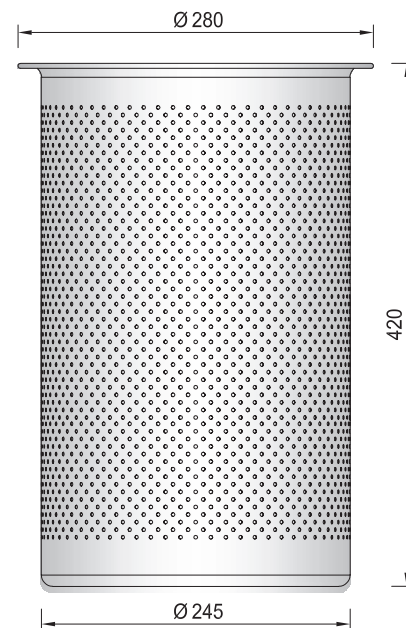
Koš za dežnike Ø245 mm, perforacija Ø3 mm
